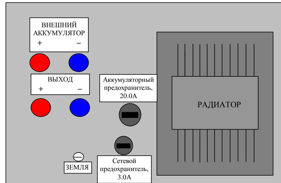
Вид сзади блока бесперебойного питания «ВОЛНА» ББП-3/20
